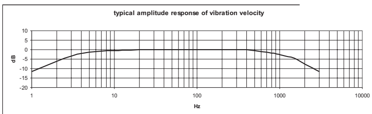
Bild Nr.1 Frequenzgang 10 Hz...1000 Hz
