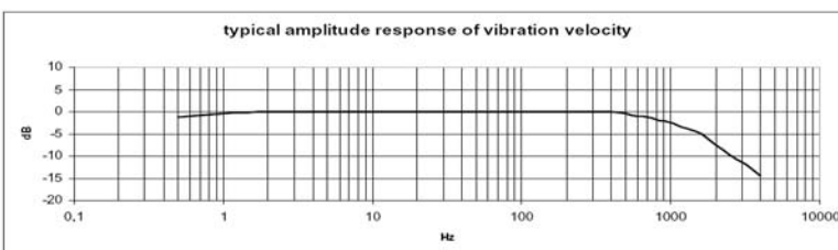
Bild Nr.2 Frequenzgang 1 Hz...1000 Hz
